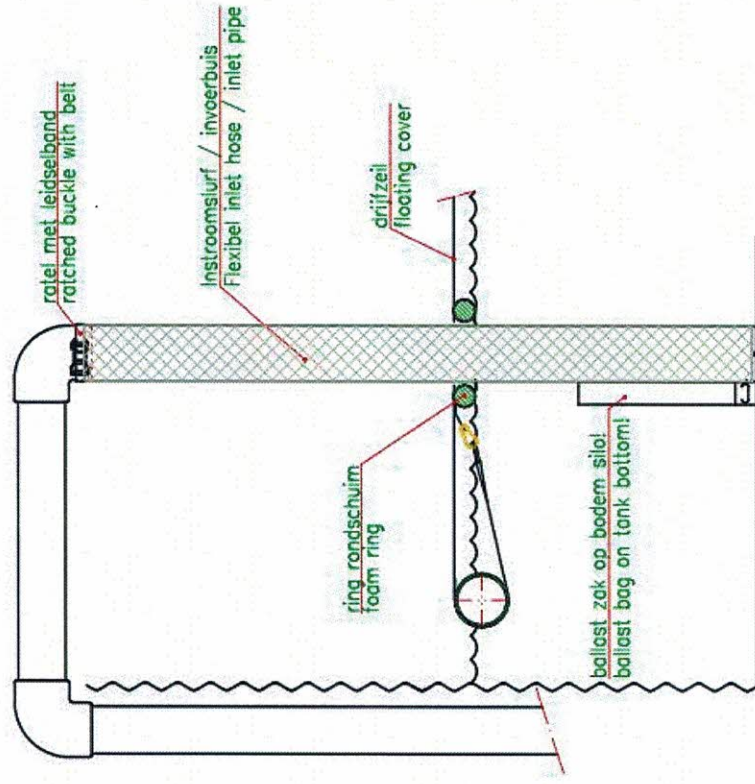
Buis inlaat / pipe inlet
