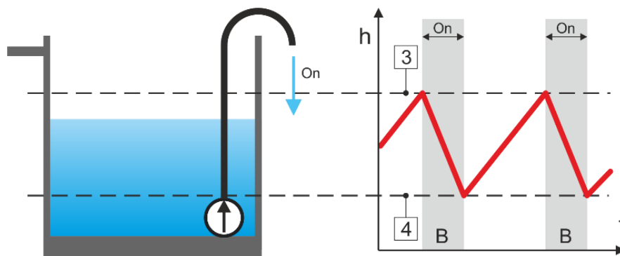
Nastavení hladiny sepnutí [3] a rozeznutí [4] pro řízené čerpání vody z jímky pomocí ponorného čerpadla
