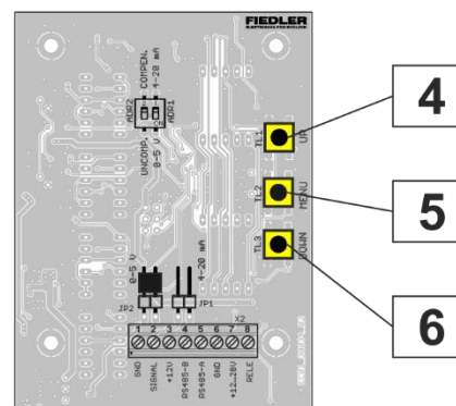
Vnitřní zadní část ovládacího panelu H520
