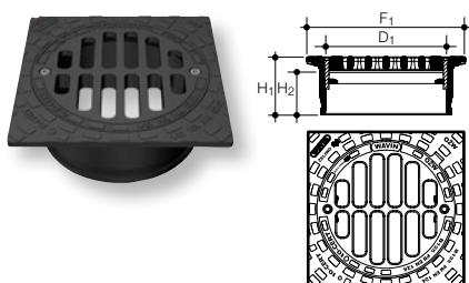
Litinná mříž B125 Ø 315 mm – do teleskopické roury
