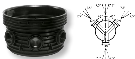
Šachtové dno Tegra 1000 NG – pro potrubí Wavin X-Stream, sběrné dno pod úhlem 45° – typ Y
