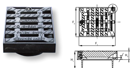
Litinná mříž D400 Ø 315 mm – do teleskopické roury
