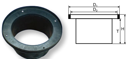
Teleskopický adaptér – pro litinové poklapy a mříže / dodáváme včetně těsnění
