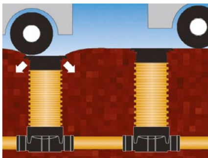
Přenos zatížení od vozidel – odolnost proti zatížení, které způsobují vozidla ve vozovce
