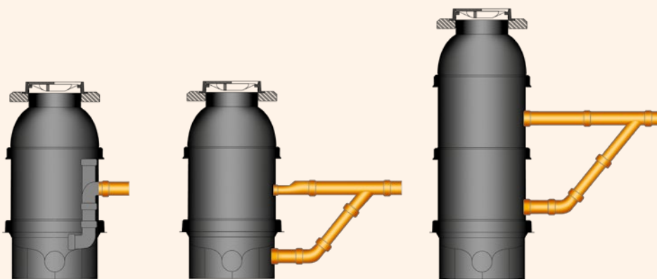
Ukázkové řešení spadišťové vstupní šachty
