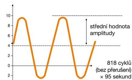
Simulace průběhu rozpínacího procesu
