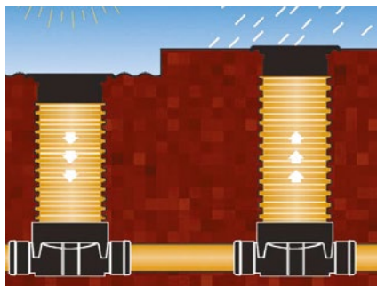
Kopírování povrchu se změnou počasí – přenos zatížení vyplývající z pohybů půdy při různém počasí a teplotě
