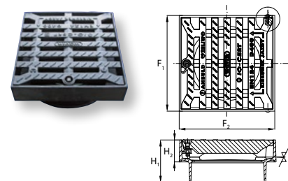
Litinná mříž D400 Ø 425 mm – do teleskopické roury
