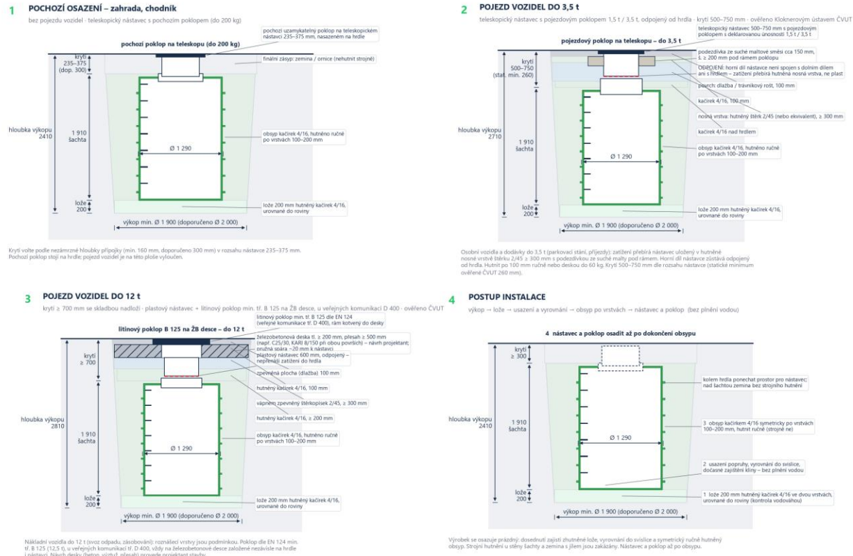
Obr. 5 – Schéma usazení DESTO-SA-1200-02 v6 (přehled).
