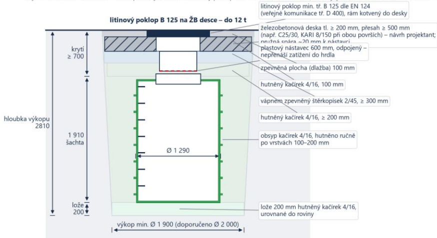
Obr. 4 – Pojezd vozidel do 12 t: krytí \geq 700 mm se skladbou nadloží, plastový nástavec, poklop min. tř. B 125 (u veřejných komunikací D 400) na železobetonové desce nezávisle na hrdle.
