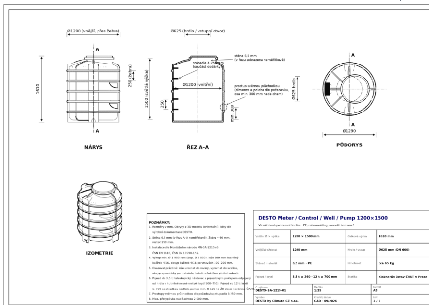
Rozměrový výkres DESTO-SA-1215-01 (nárys, řez A-A, půdorys). PDF + DXF ke stažení.
